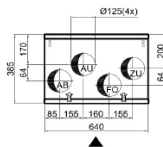
EA180.6 Bypass rechts
