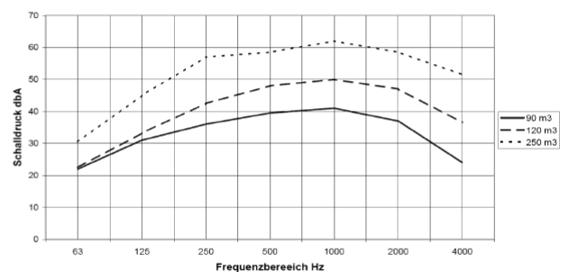
Schallwerte im Zuluftkanal EuroAir 250
